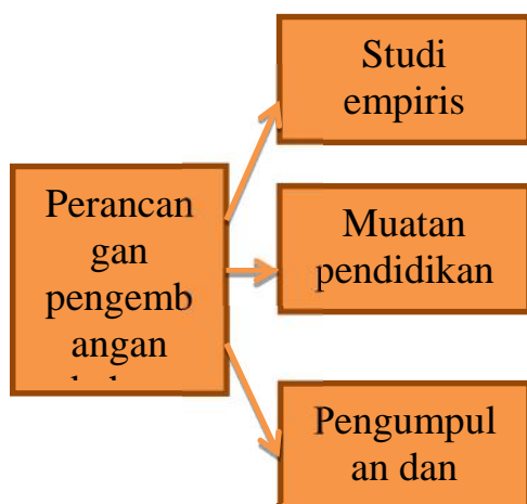
Gambar 3.1. Langkah-langkah Penelitian
